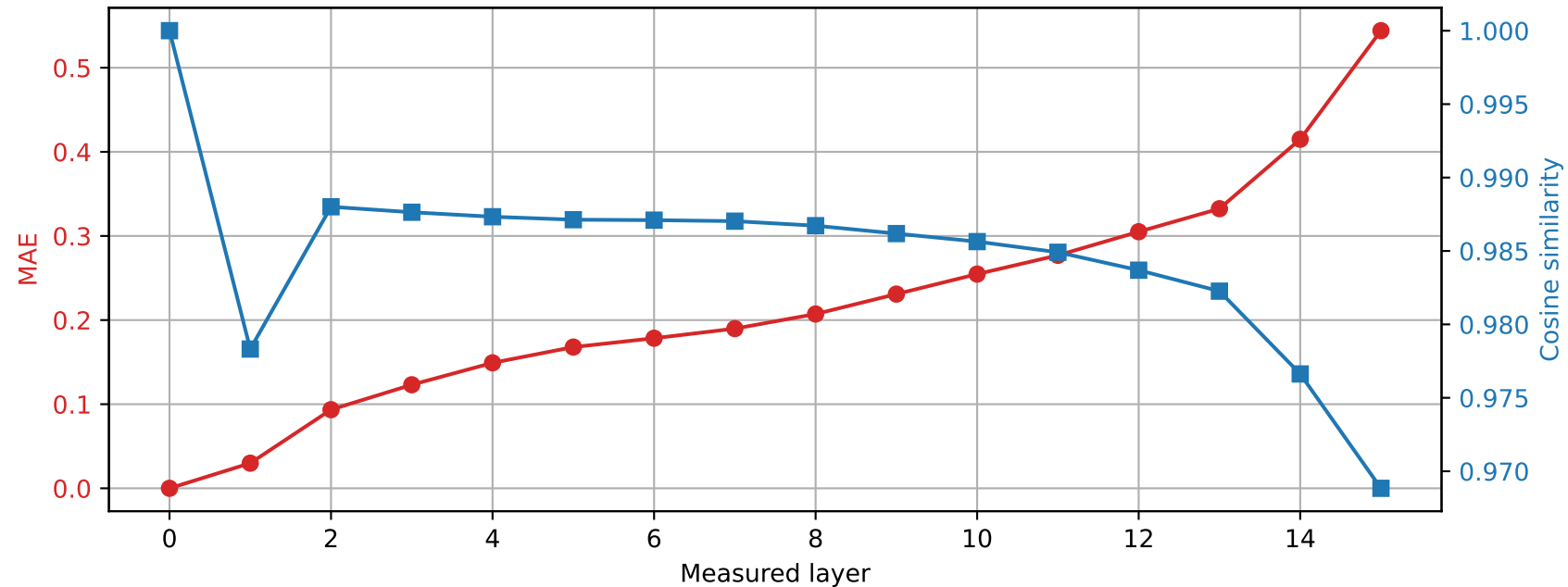
Llama-3.2-1B | Prompt 1 Spared layer 10 | Hybrid vs unquantized
