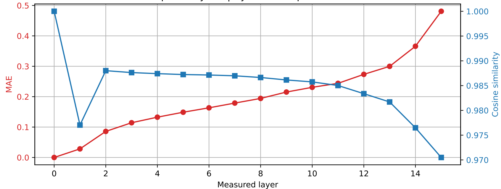
Llama-3.2-1B | Prompt 2 Spared layer 7 | Hybrid vs unquantized
