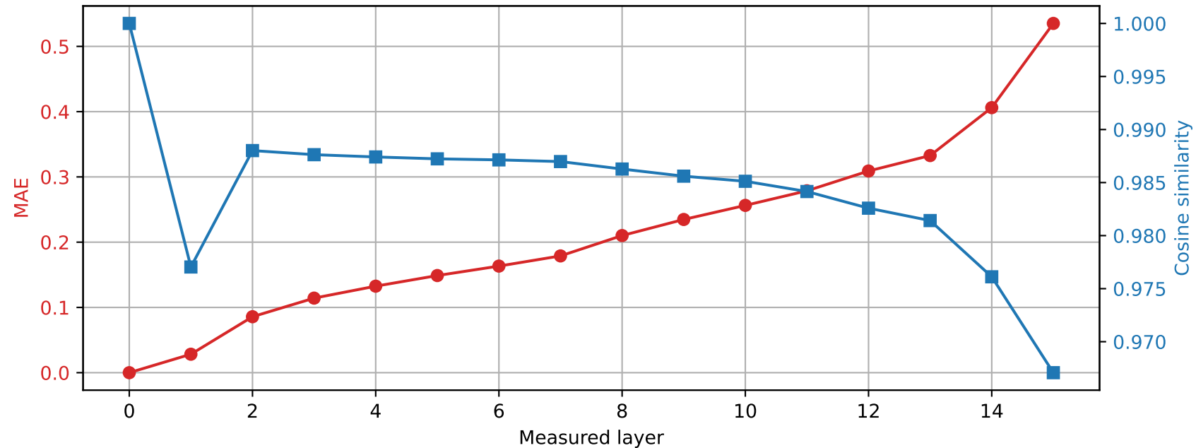
Llama-3.2-1B | Prompt 2 Spared layer 10 | Hybrid vs unquantized
