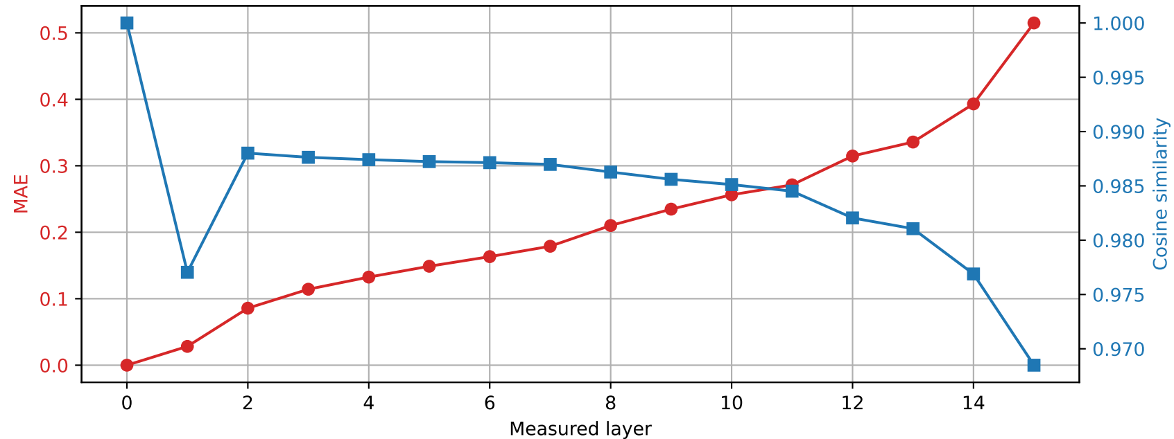
Llama-3.2-1B | Prompt 2 Spared layer 11 | Hybrid vs unquantized
