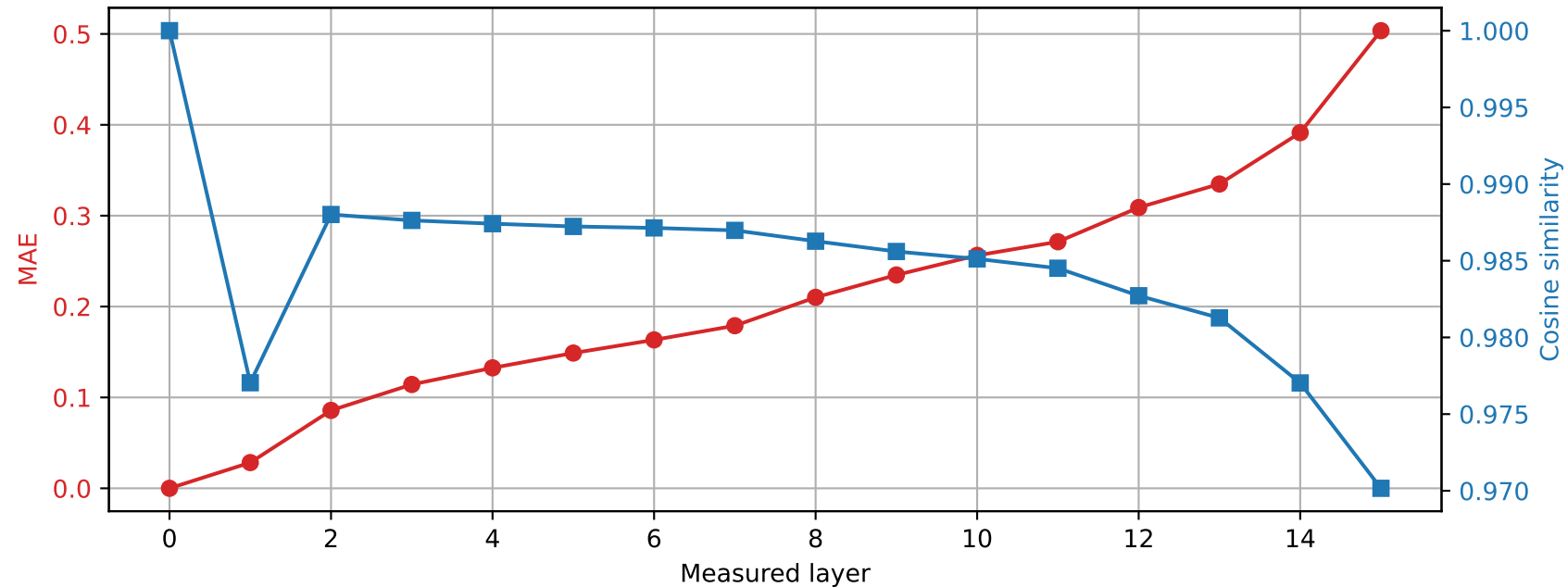
Llama-3.2-1B | Prompt 2 Spared layer 13 | Hybrid vs unquantized
