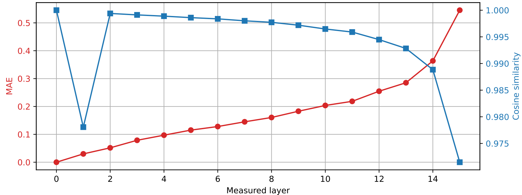
Llama-3.2-1B | Prompt 3 Spared layer 1 | Hybrid vs unquantized
