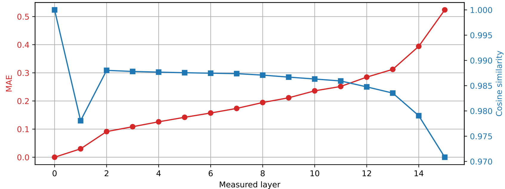
Llama-3.2-1B | Prompt 3 Spared layer 2 | Hybrid vs unquantized
