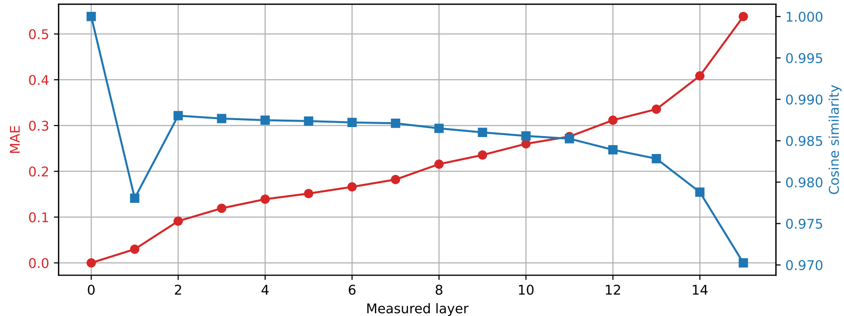
Llama-3.2-1B | Prompt 3 Spared layer 4 | Hybrid vs unquantized
