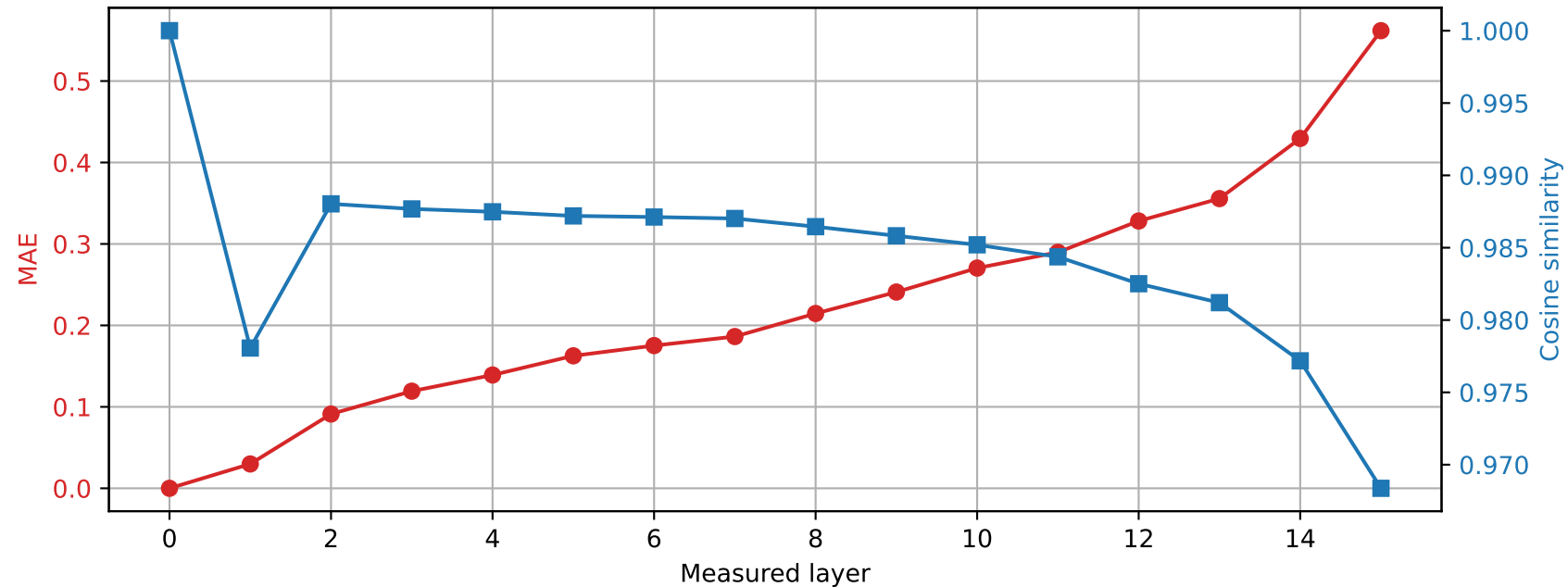
Llama-3.2-1B | Prompt 3 Spared layer 6 | Hybrid vs unquantized
