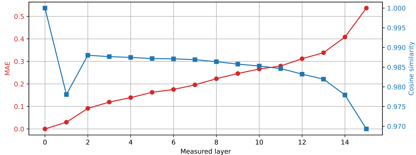
Llama-3.2-1B | Prompt 3 Spared layer 7 | Hybrid vs unquantized
