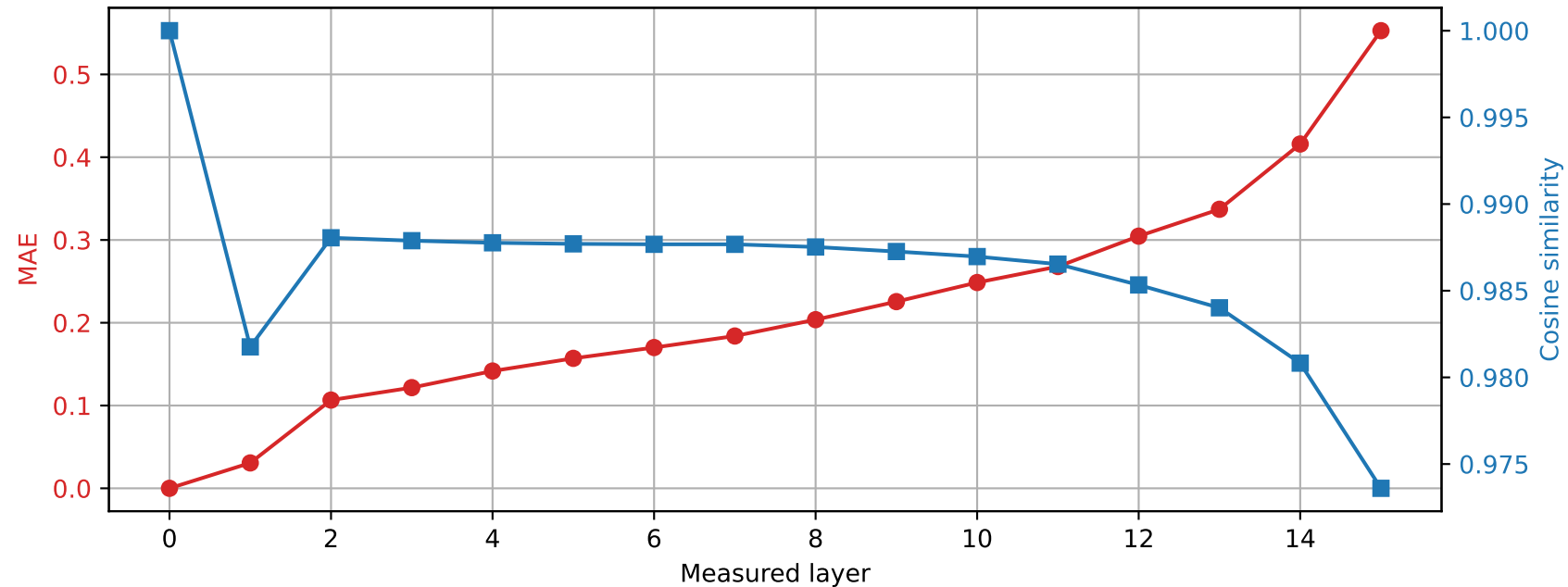
Llama-3.2-1B | Prompt 4 Spared layer 2 | Hybrid vs unquantized
