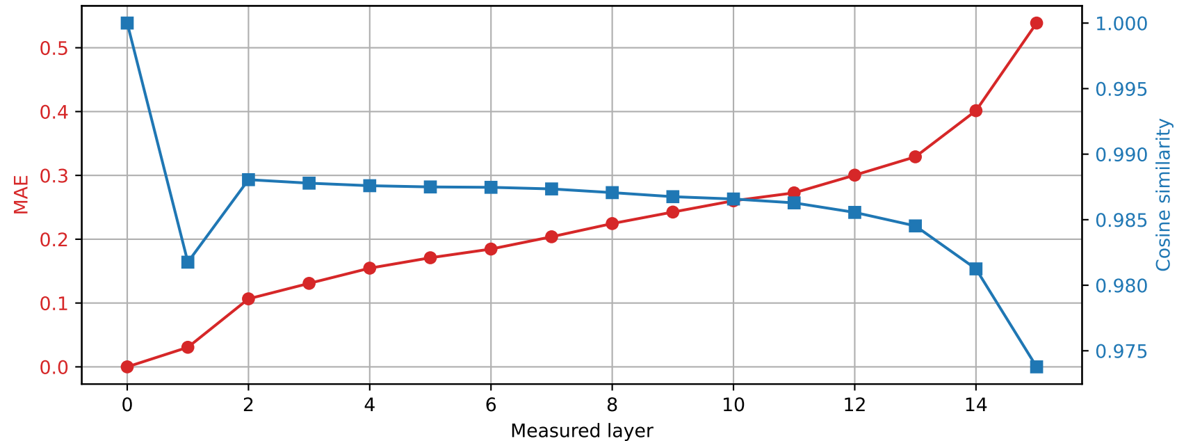
Llama-3.2-1B | Prompt 4 Spared layer 8 | Hybrid vs unquantized
