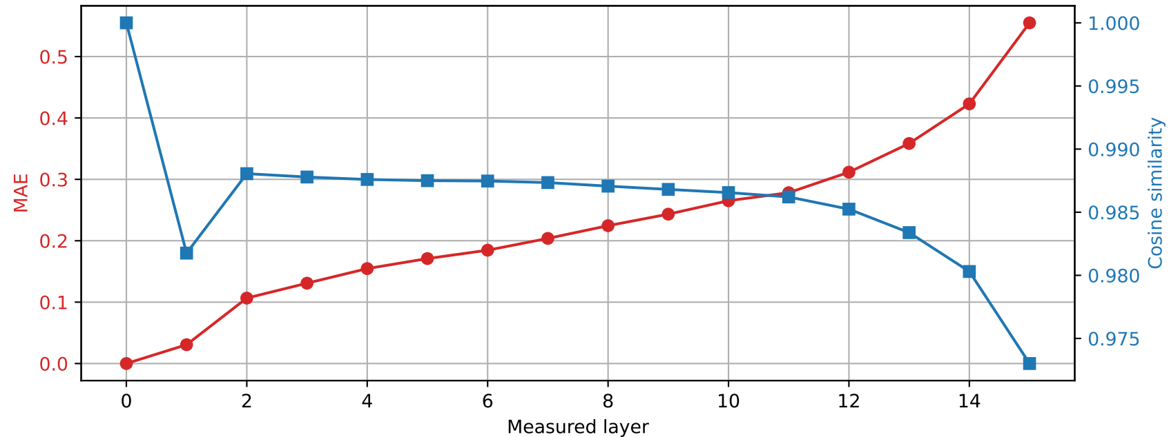
Llama-3.2-1B | Prompt 4 Spared layer 12 | Hybrid vs unquantized
