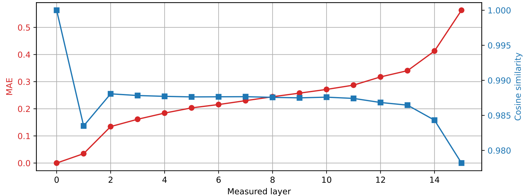
Llama-3.2-1B | Prompt 0 Spared layer 7 | Hybrid vs unquantized
