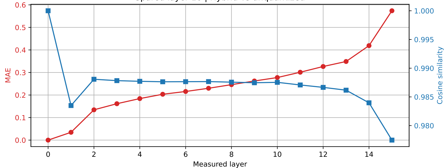
Llama-3.2-1B | Prompt 0 Spared layer 10 | Hybrid vs unquantized
