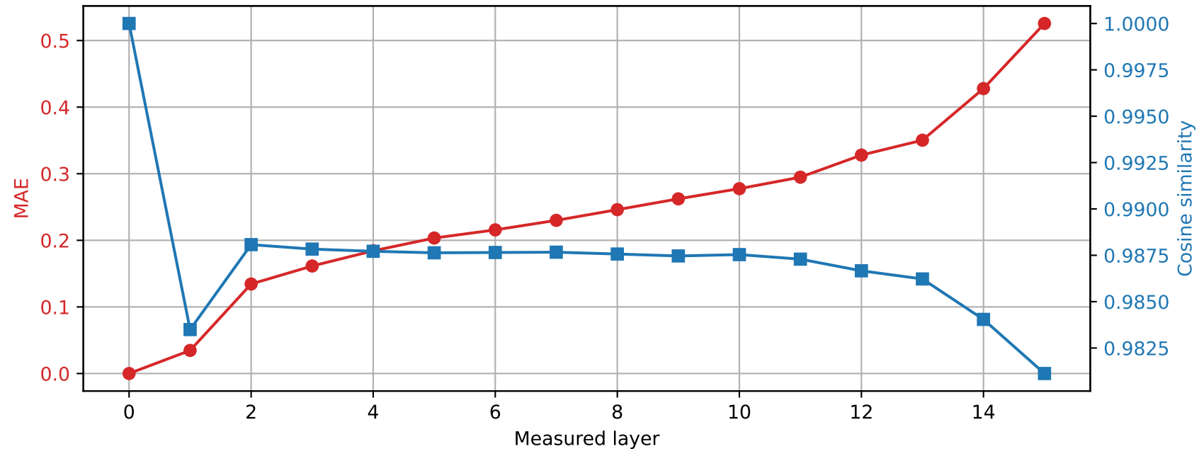
Llama-3.2-1B | Prompt 0 Spared layer 14 | Hybrid vs unquantized
