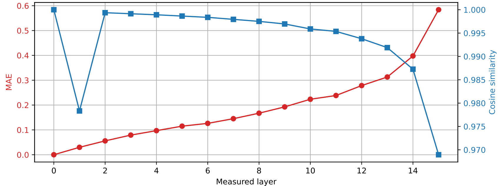
Llama-3.2-1B | Prompt 1 Spared layer 1 | Hybrid vs unquantized
