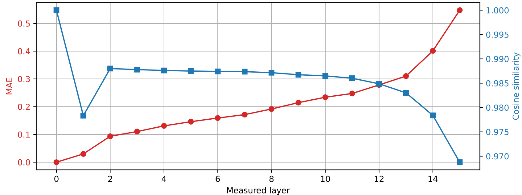
Llama-3.2-1B | Prompt 1 Spared layer 2 | Hybrid vs unquantized
