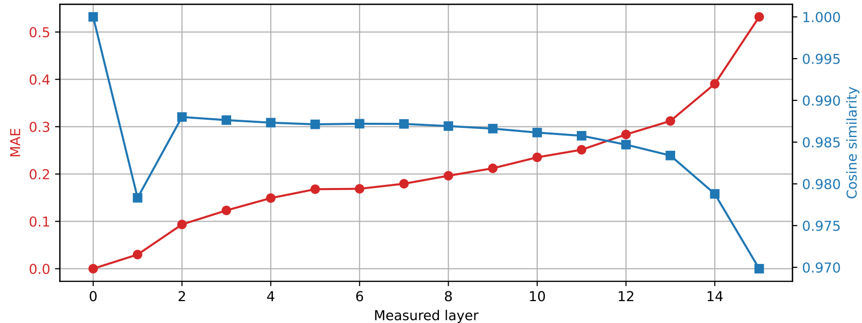
Llama-3.2-1B | Prompt 1 Spared layer 5 | Hybrid vs unquantized
