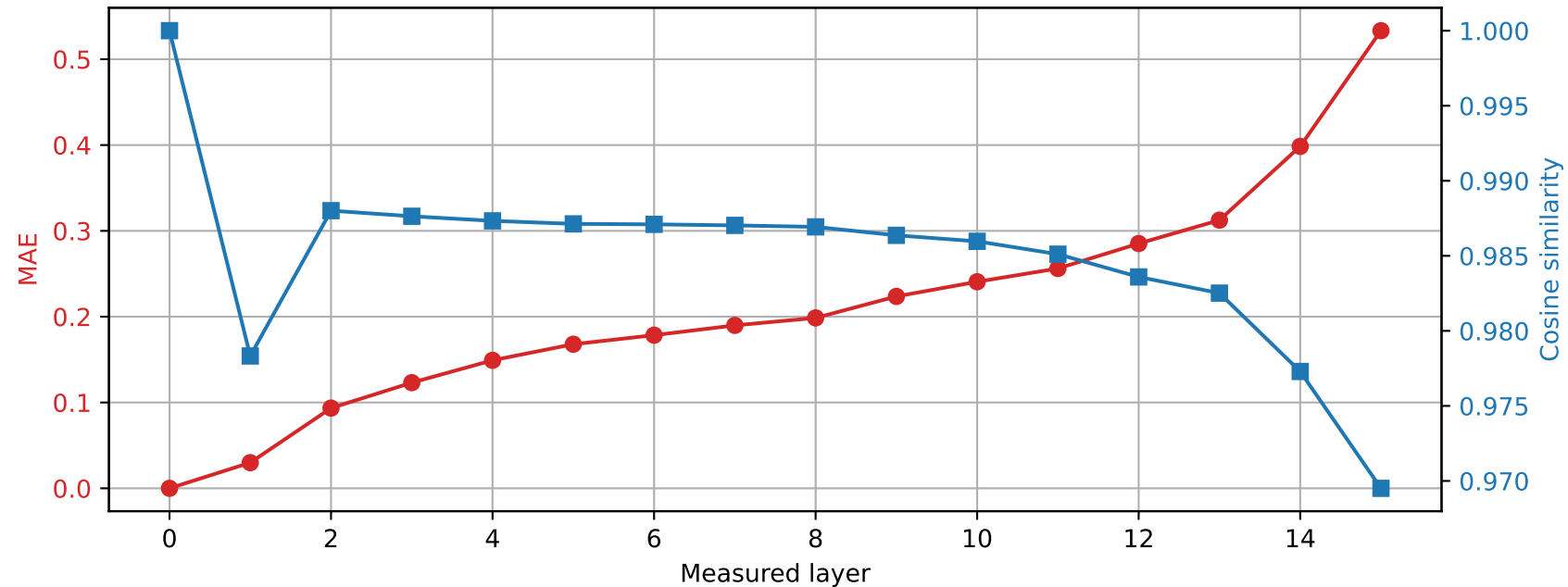
Llama-3.2-1B | Prompt 1 Spared layer 7 | Hybrid vs unquantized
