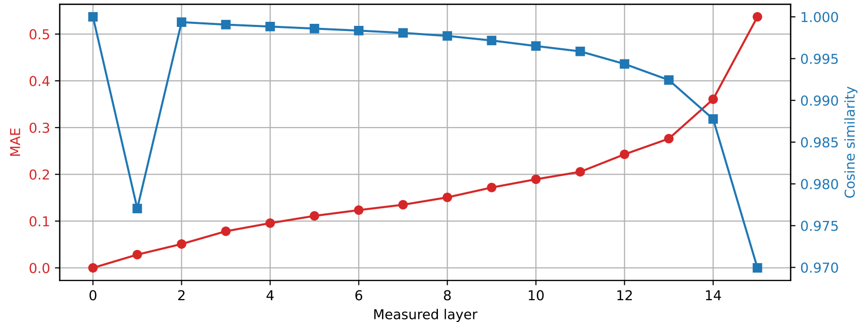
Llama-3.2-1B | Prompt 2 Spared layer 1 | Hybrid vs unquantized
