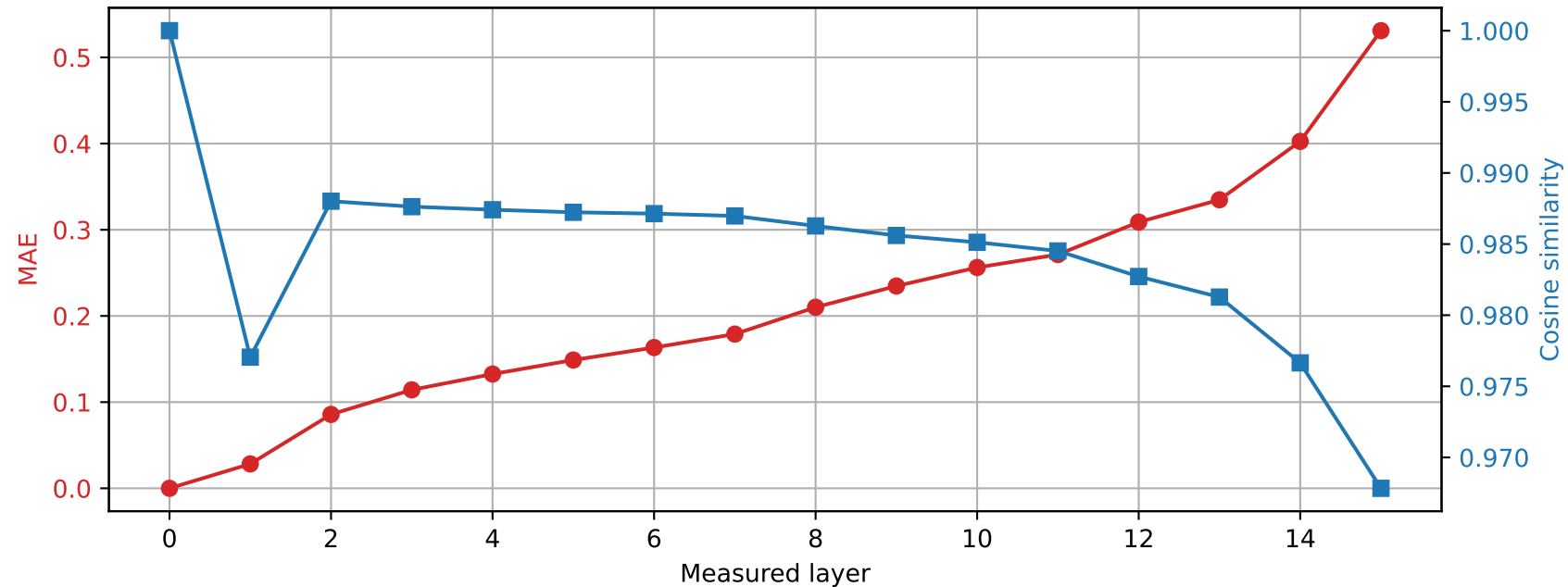
Llama-3.2-1B | Prompt 2 Spared layer 15 | Hybrid vs unquantized
