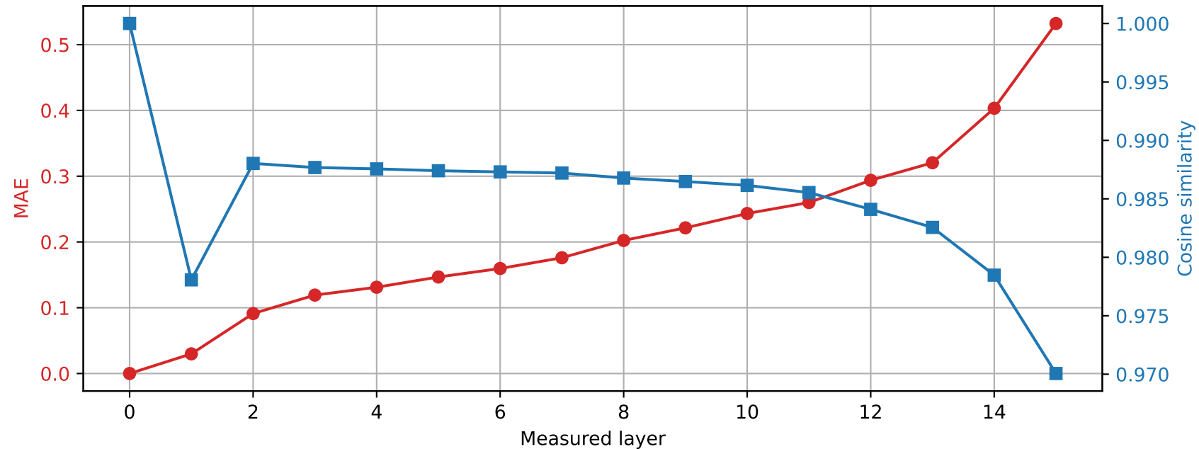
Llama-3.2-1B | Prompt 3 Spared layer 3 | Hybrid vs unquantized
