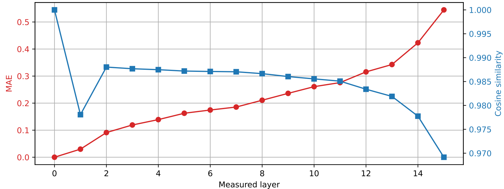
Llama-3.2-1B | Prompt 3 Spared layer 5 | Hybrid vs unquantized
