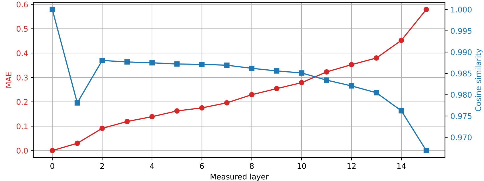
Llama-3.2-1B | Prompt 3 Spared layer 10 | Hybrid vs unquantized
