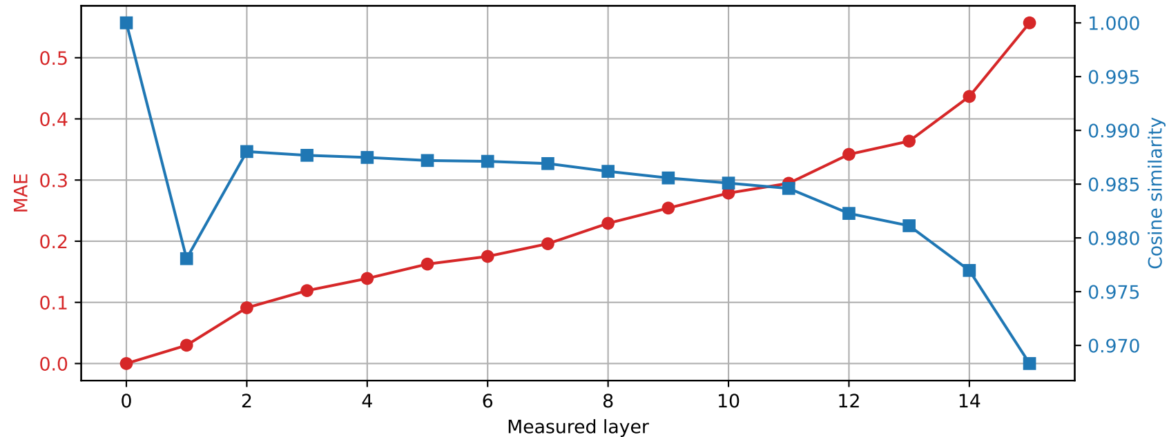
Llama-3.2-1B | Prompt 3 Spared layer 11 | Hybrid vs unquantized
