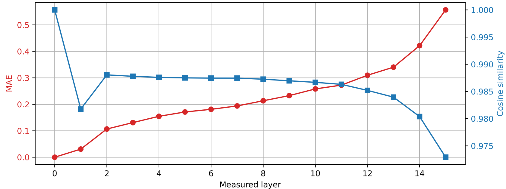
Llama-3.2-1B | Prompt 4 Spared layer 5 | Hybrid vs unquantized
