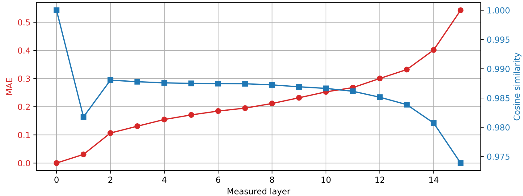
Llama-3.2-1B | Prompt 4 Spared layer 6 | Hybrid vs unquantized
