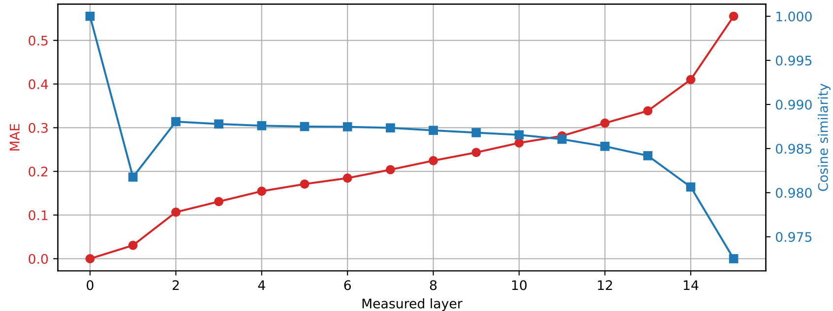
Llama-3.2-1B | Prompt 4 Spared layer 10 | Hybrid vs unquantized
