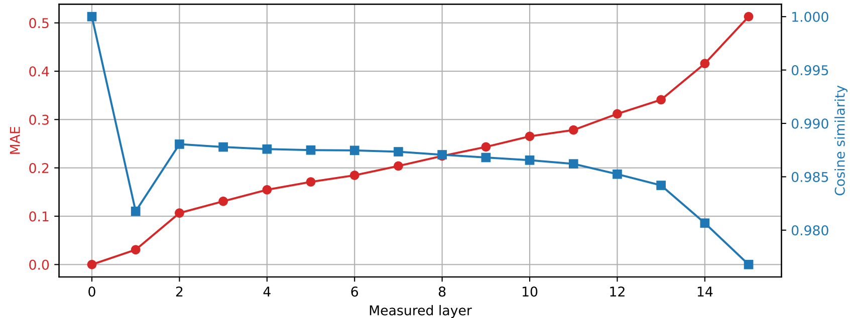
Llama-3.2-1B | Prompt 4 Spared layer 14 | Hybrid vs unquantized
