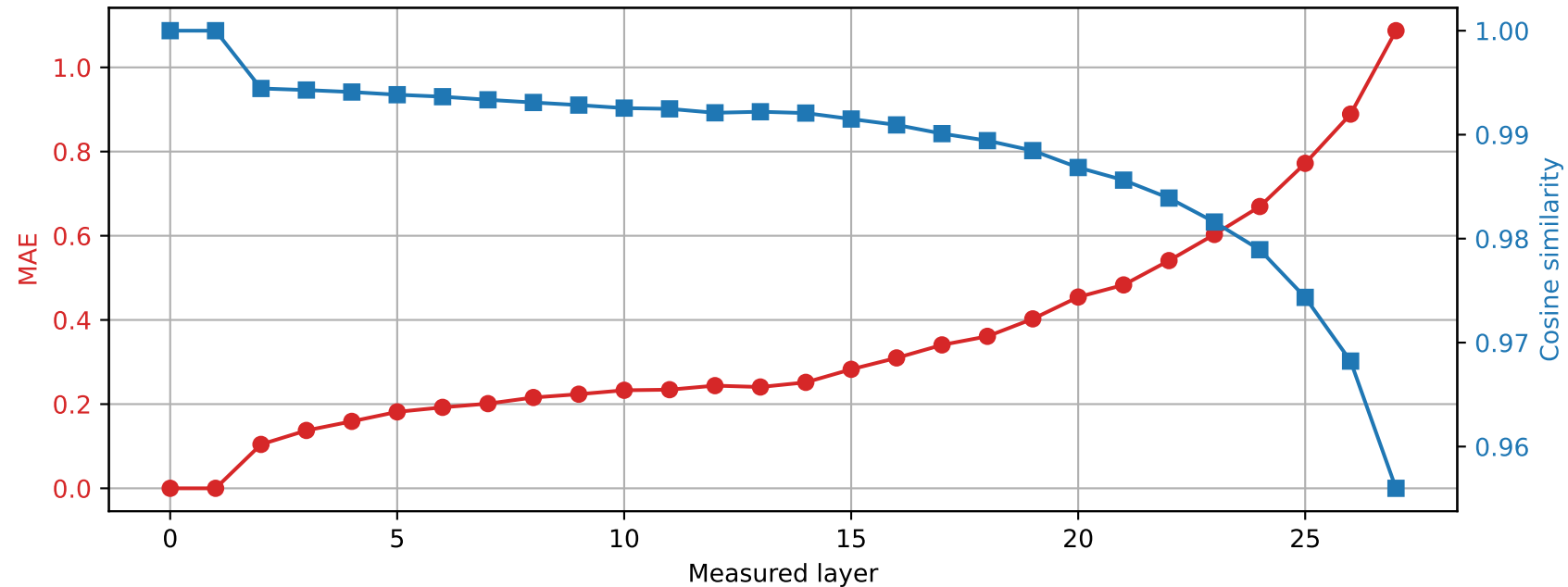
Llama-3.2-3B | Prompt 0 Spared layer 0 | Hybrid vs unquantized
