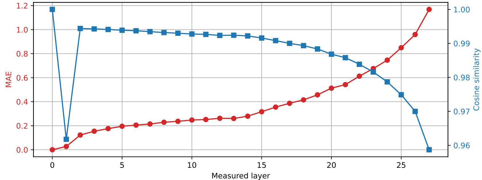
Llama-3.2-3B | Prompt 0 Spared layer 3 | Hybrid vs unquantized
