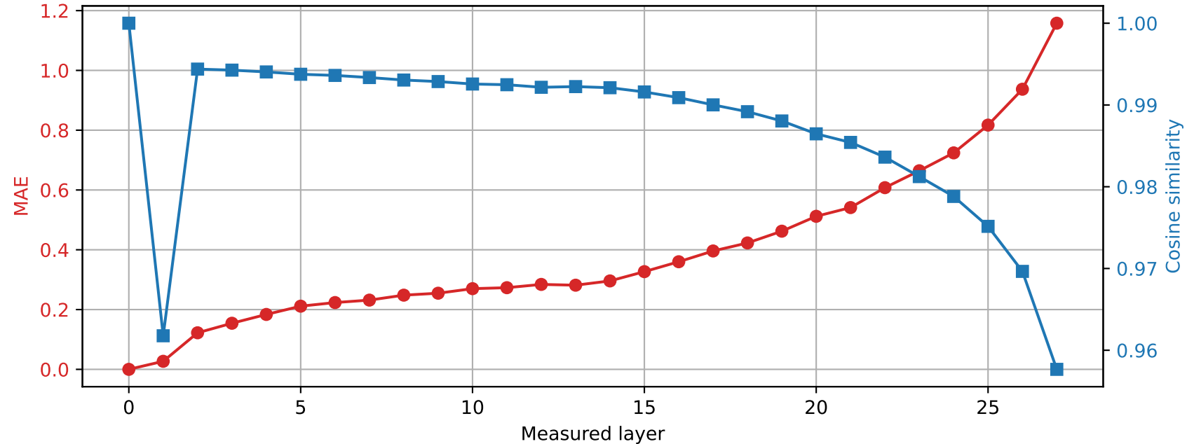
Llama-3.2-3B | Prompt 0 Spared layer 5 | Hybrid vs unquantized
