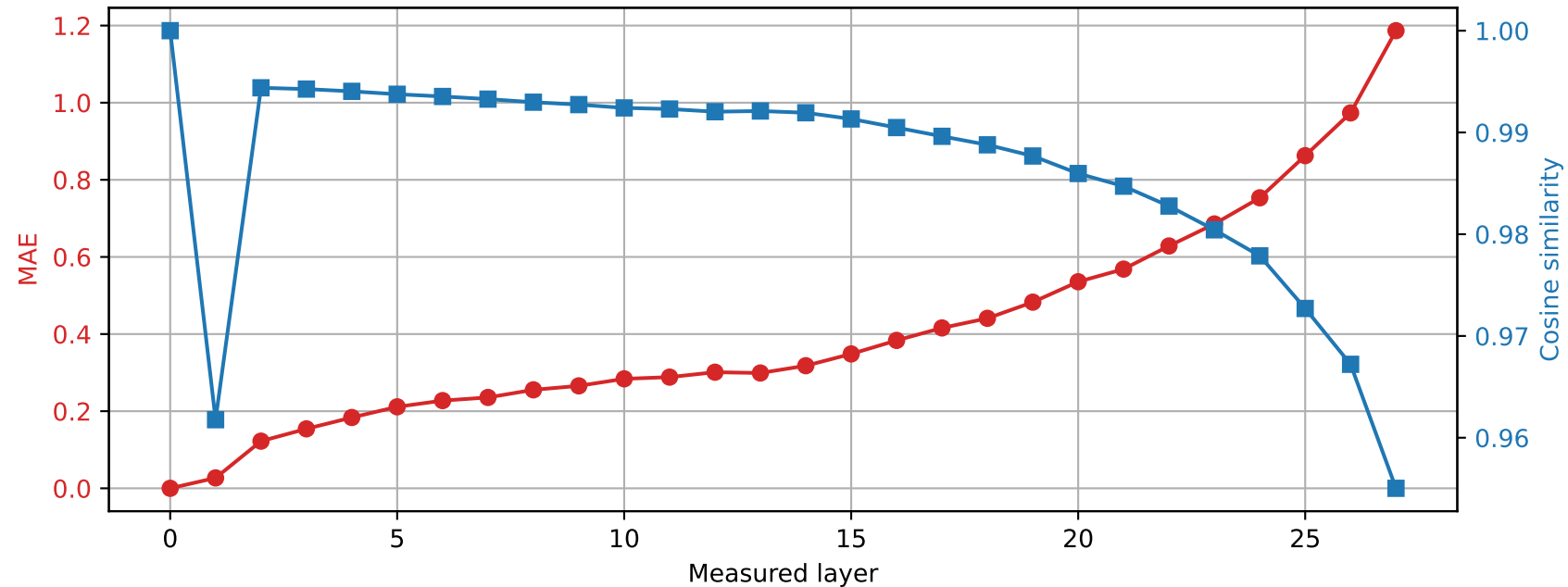
Llama-3.2-3B | Prompt 0 Spared layer 11 | Hybrid vs unquantized
