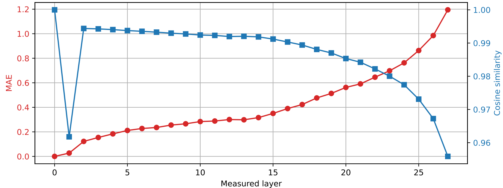
Llama-3.2-3B | Prompt 0 Spared layer 17 | Hybrid vs unquantized
