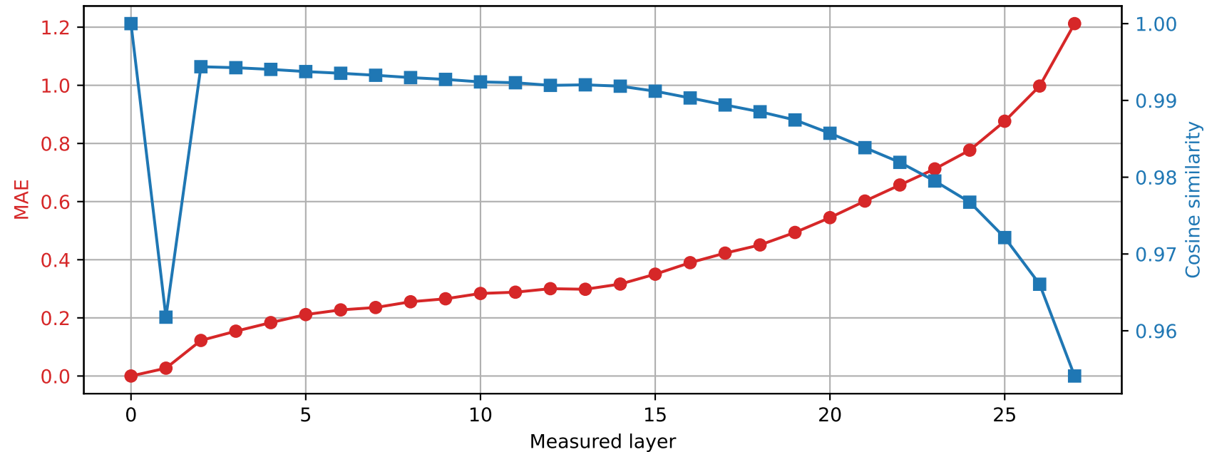
Llama-3.2-3B | Prompt 0 Spared layer 20 | Hybrid vs unquantized
