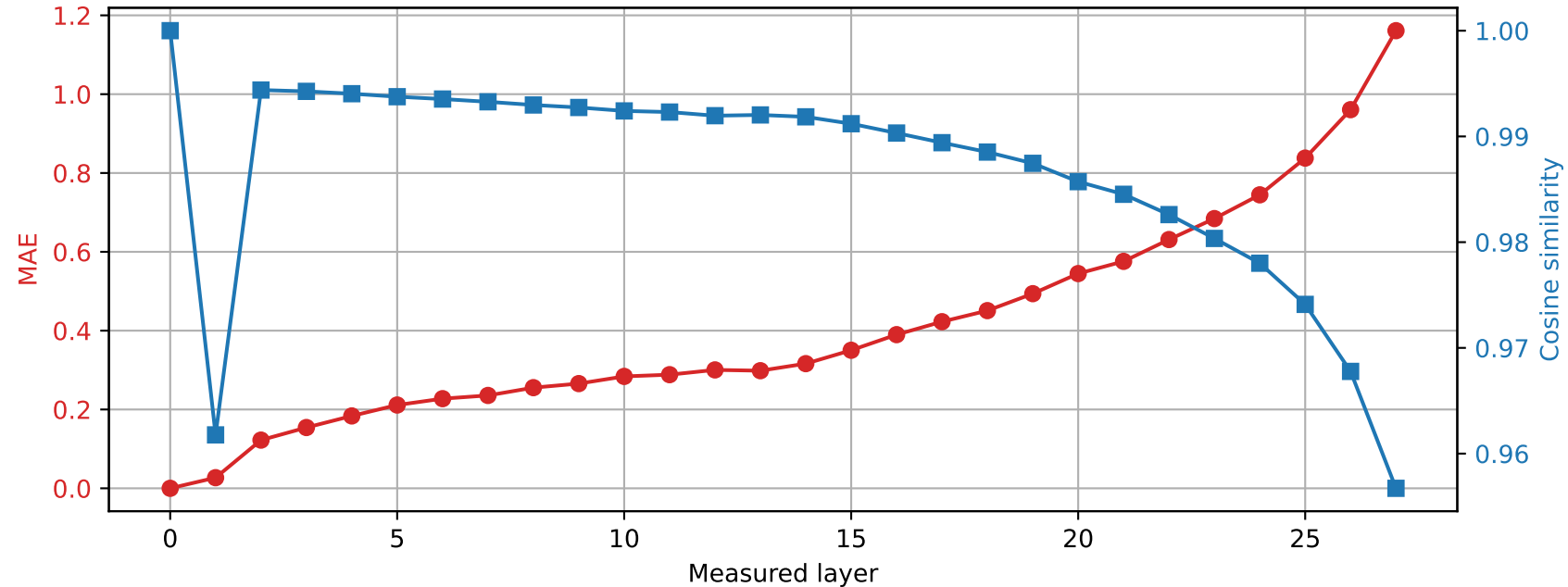
Llama-3.2-3B | Prompt 0 Spared layer 22 | Hybrid vs unquantized
