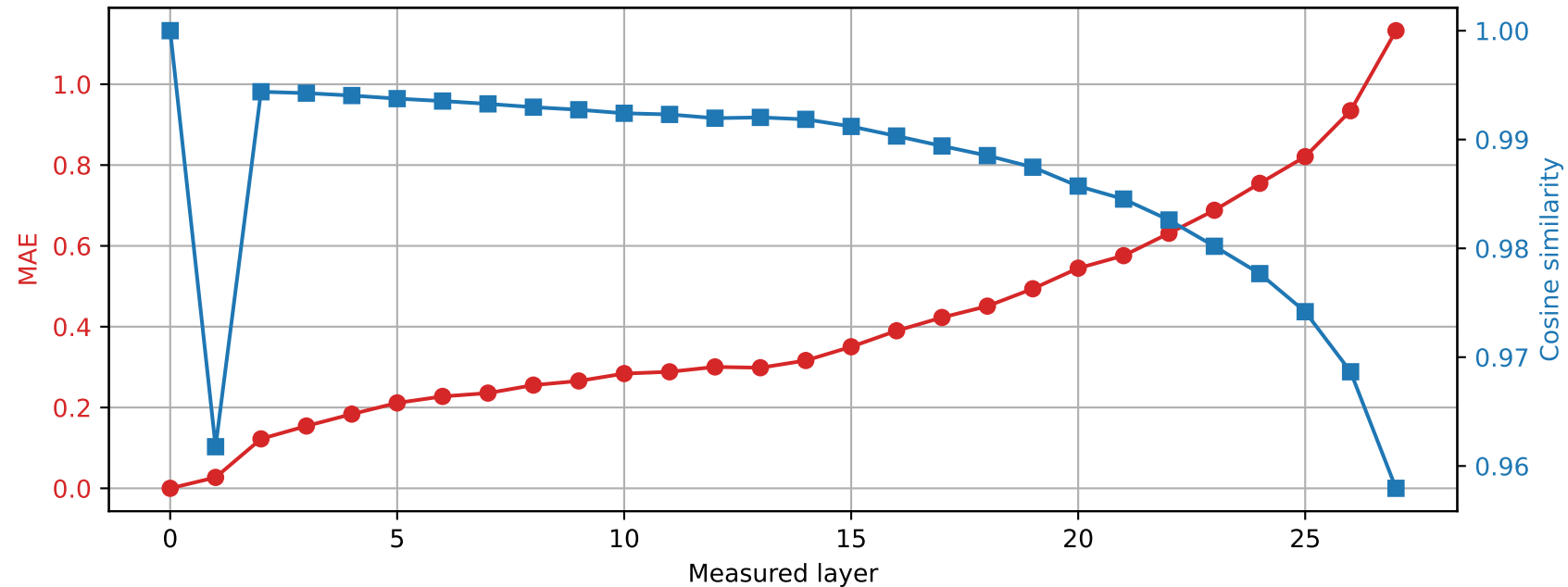
Llama-3.2-3B | Prompt 0 Spared layer 24 | Hybrid vs unquantized
