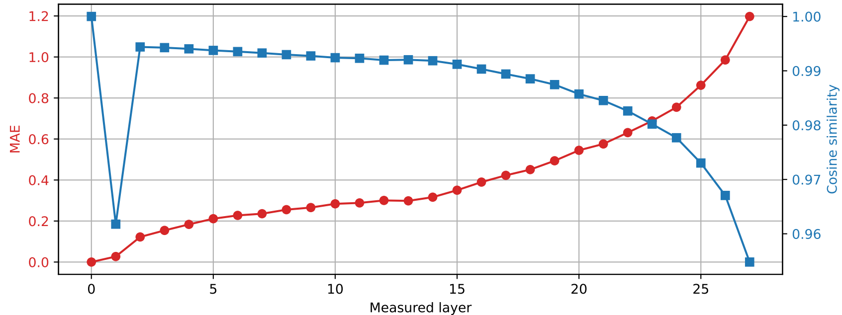
Llama-3.2-3B | Prompt 0 Spared layer 27 | Hybrid vs unquantized
