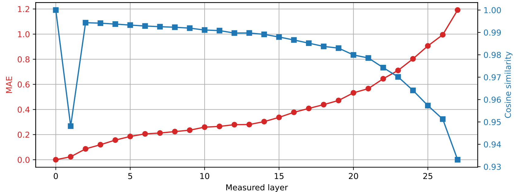
Llama-3.2-3B | Prompt 1 Spared layer 7 | Hybrid vs unquantized
