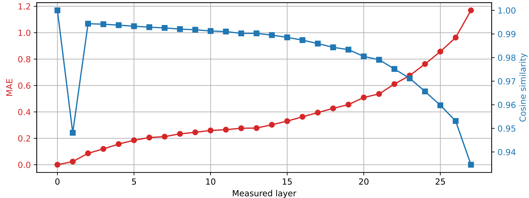
Llama-3.2-3B | Prompt 1 Spared layer 8 | Hybrid vs unquantized
