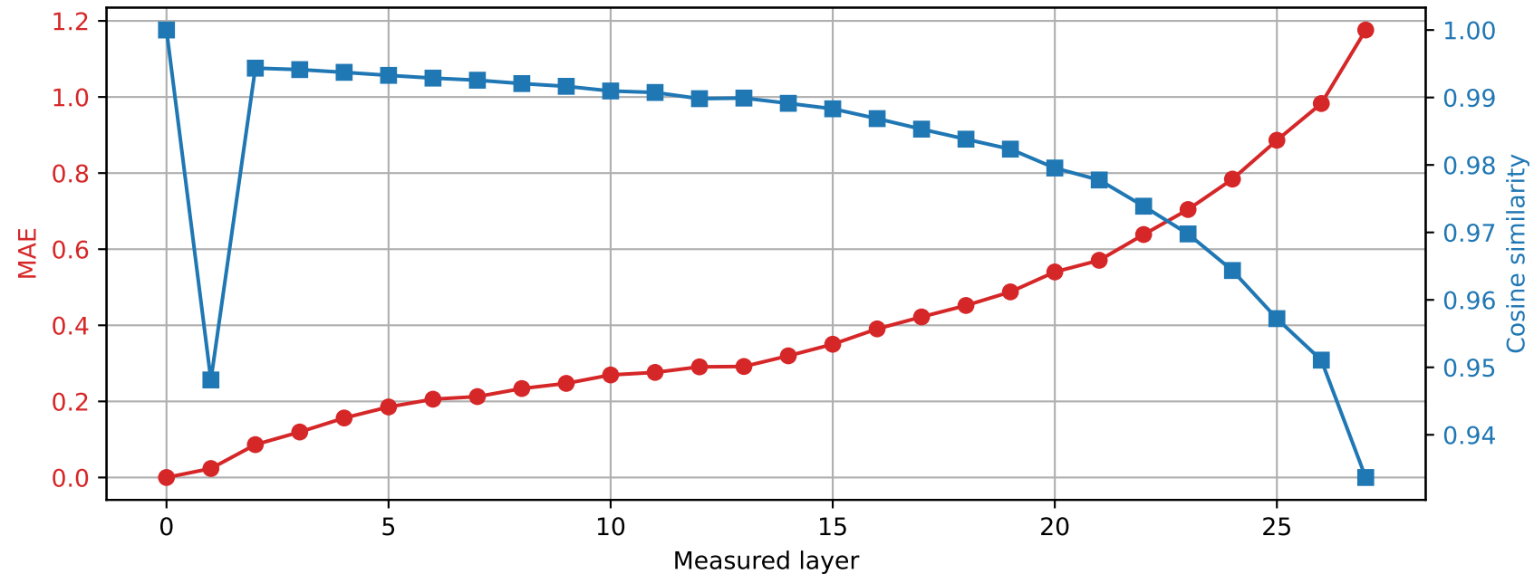
Llama-3.2-3B | Prompt 1 Spared layer 14 | Hybrid vs unquantized
