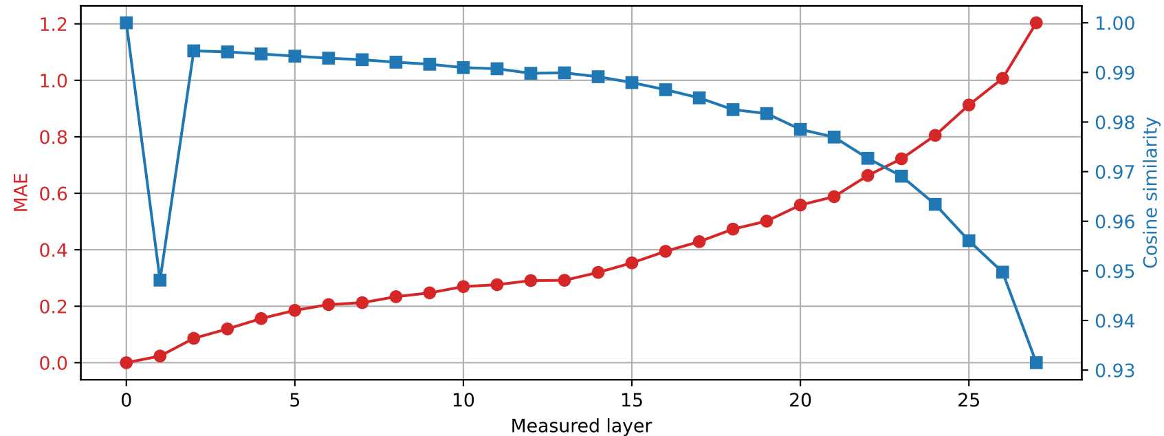
Llama-3.2-3B | Prompt 1 Spared layer 17 | Hybrid vs unquantized
