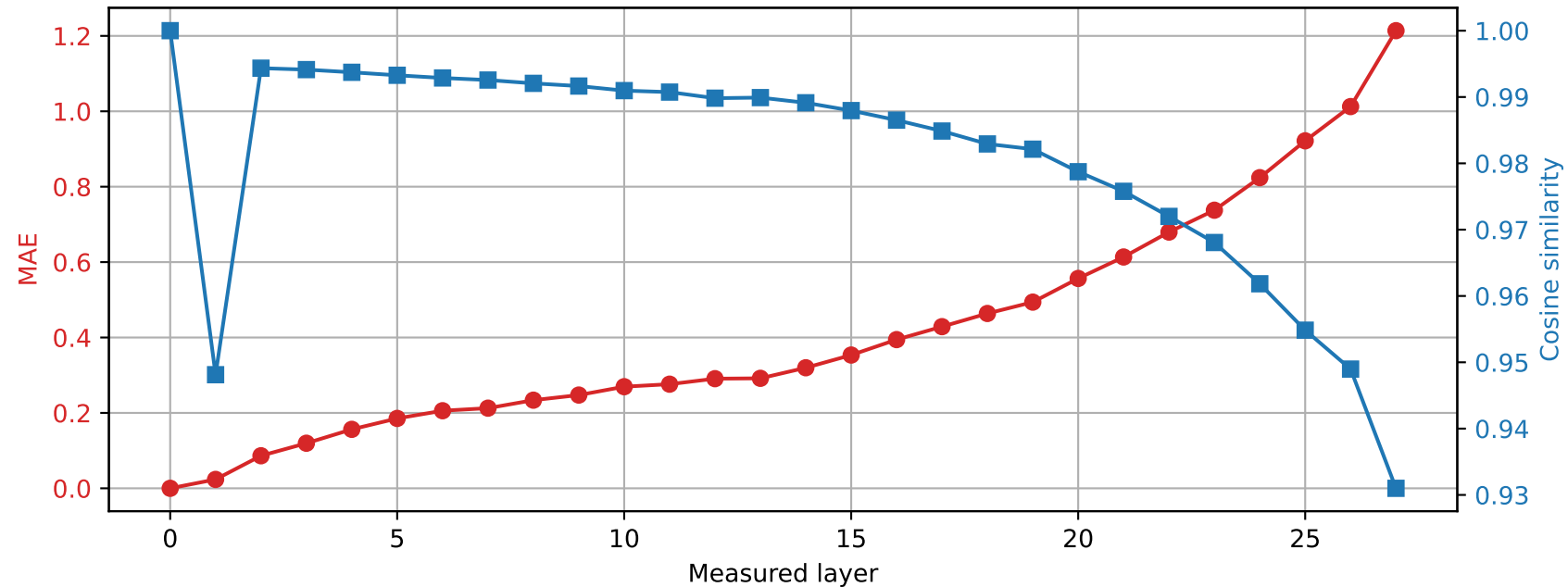
Llama-3.2-3B | Prompt 1 Spared layer 20 | Hybrid vs unquantized
