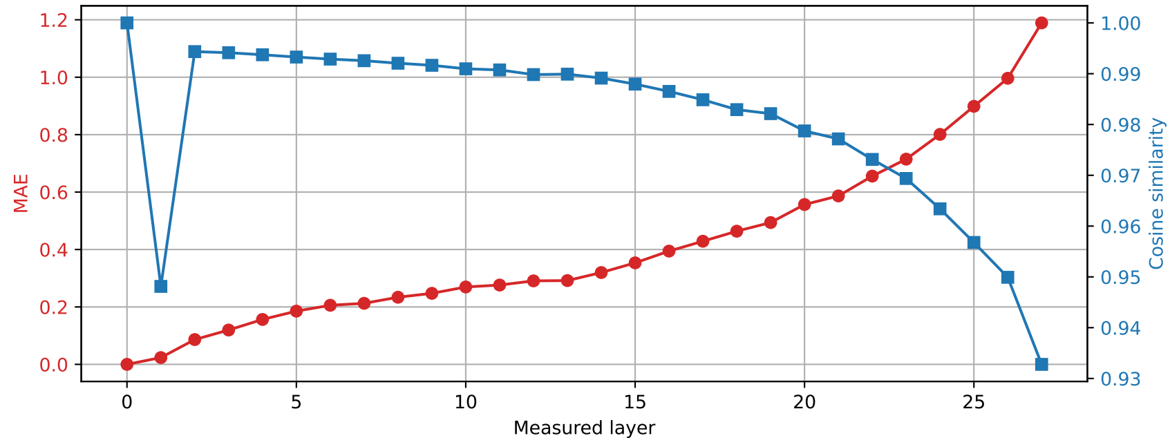
Llama-3.2-3B | Prompt 1 Spared layer 22 | Hybrid vs unquantized
