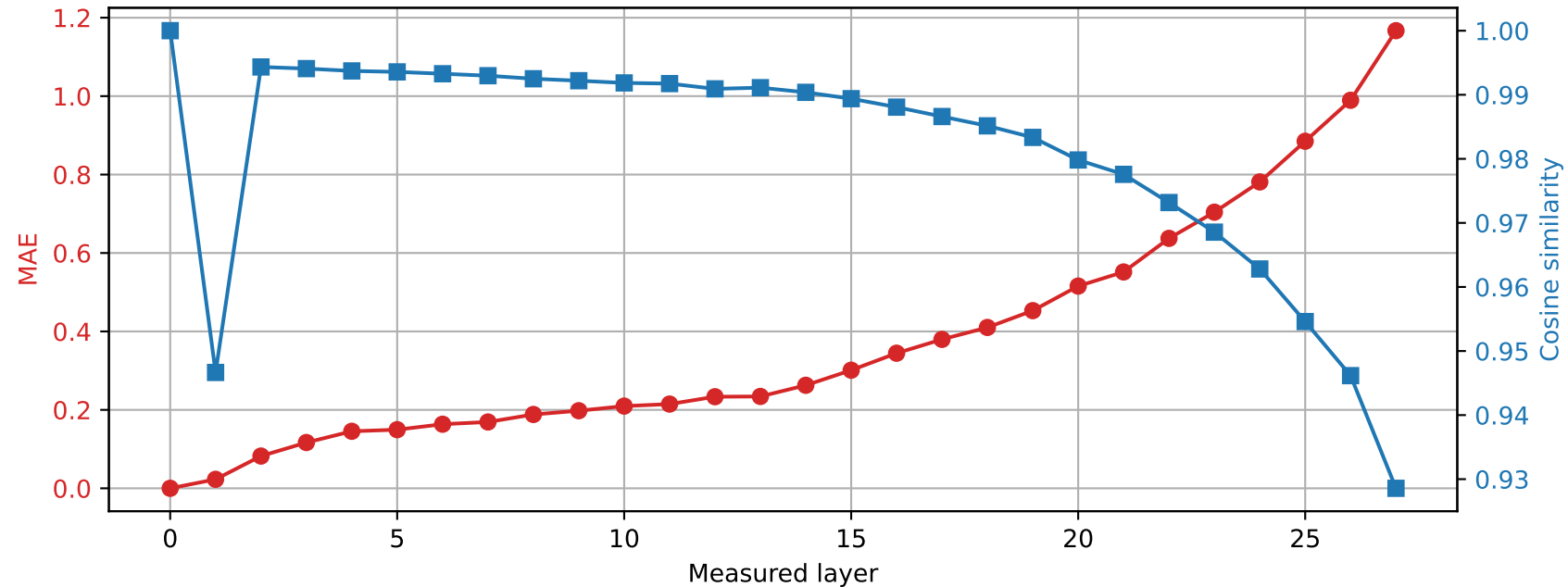
Llama-3.2-3B | Prompt 2 Spared layer 4 | Hybrid vs unquantized
