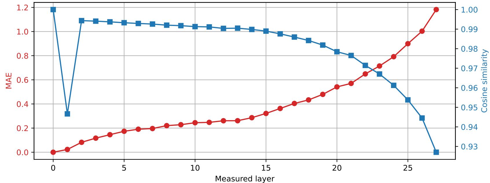
Llama-3.2-3B | Prompt 2 Spared layer 8 | Hybrid vs unquantized
