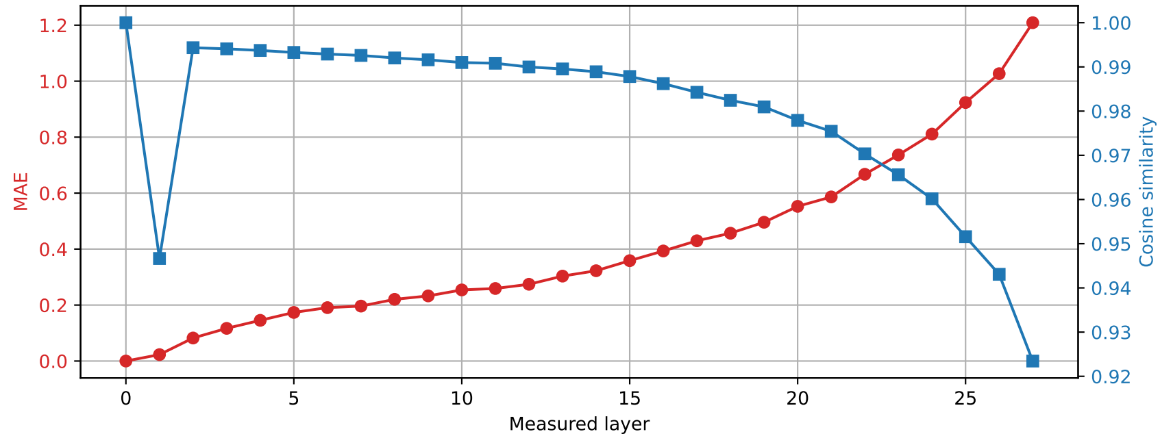
Llama-3.2-3B | Prompt 2 Spared layer 12 | Hybrid vs unquantized
