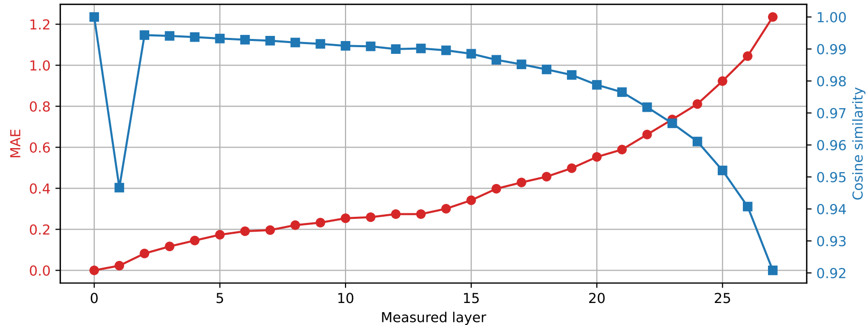
Llama-3.2-3B | Prompt 2 Spared layer 15 | Hybrid vs unquantized
