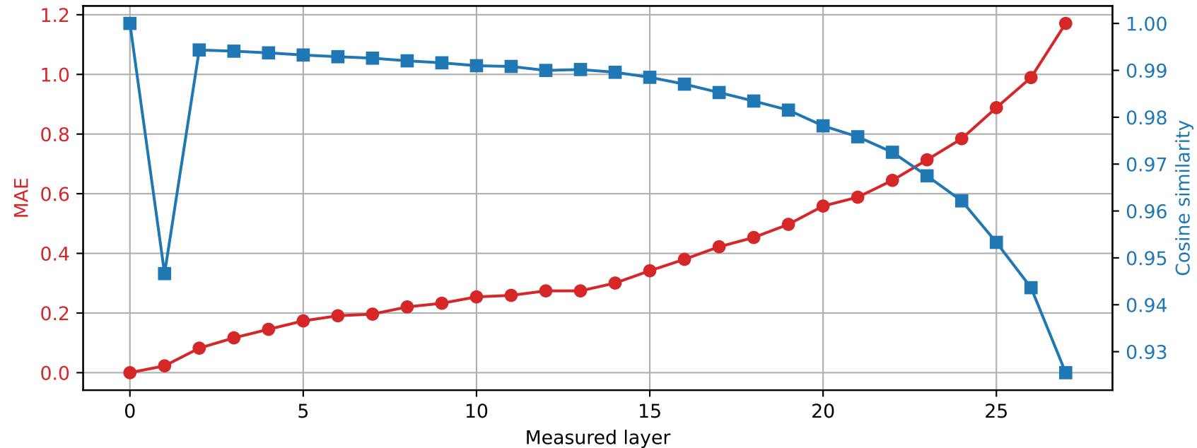
Llama-3.2-3B | Prompt 2 Spared layer 21 | Hybrid vs unquantized
